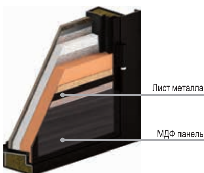
Вид в разрезе
